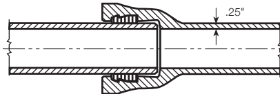
A-703 2"
