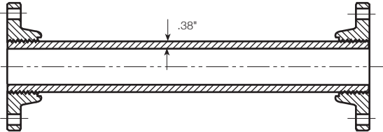
A-706 2"
