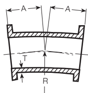
A-506 11¼° Bend
