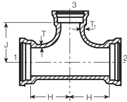
A-214 All Bell Tee
