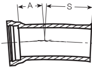
A-107 Bell & Spigot 11 1/4° Bend
