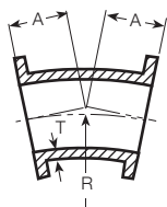
A-504 22½° Bend
